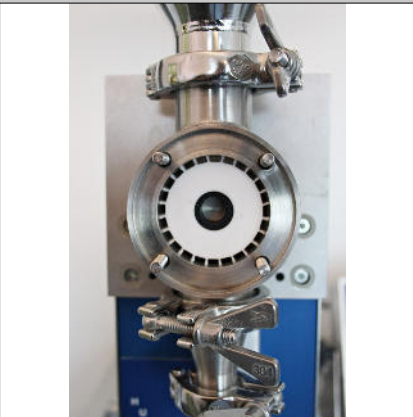
VAM-Abfüllköpfe VAM-fillingheads
